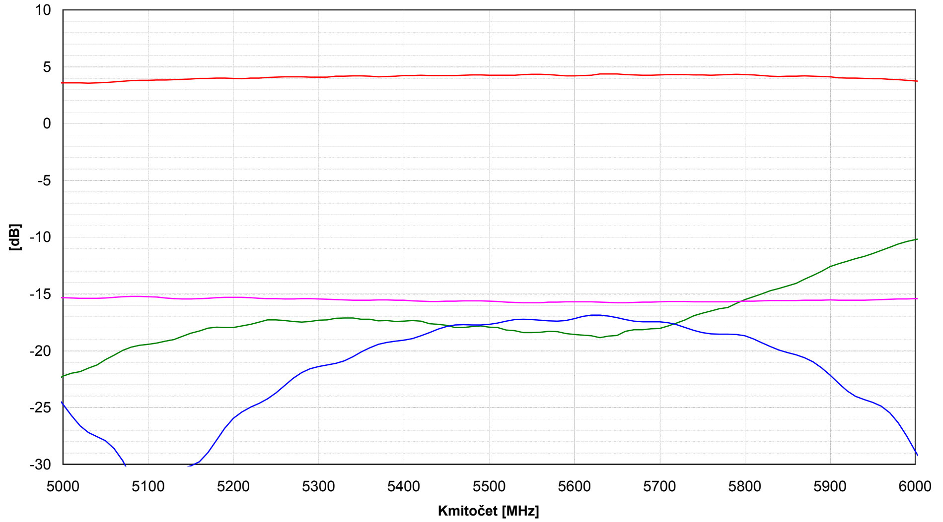
ADA 16 - S parametry
